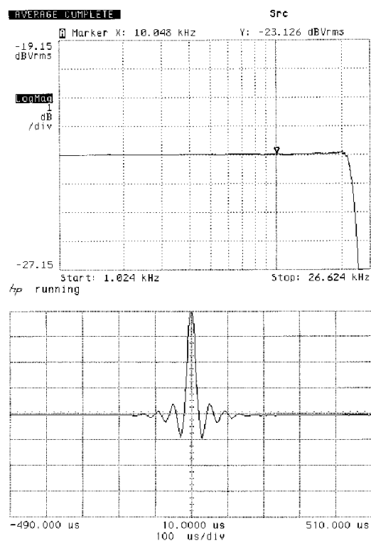
短程 (有限脉冲响应) 滤波器的频率响应和瞬态特性
