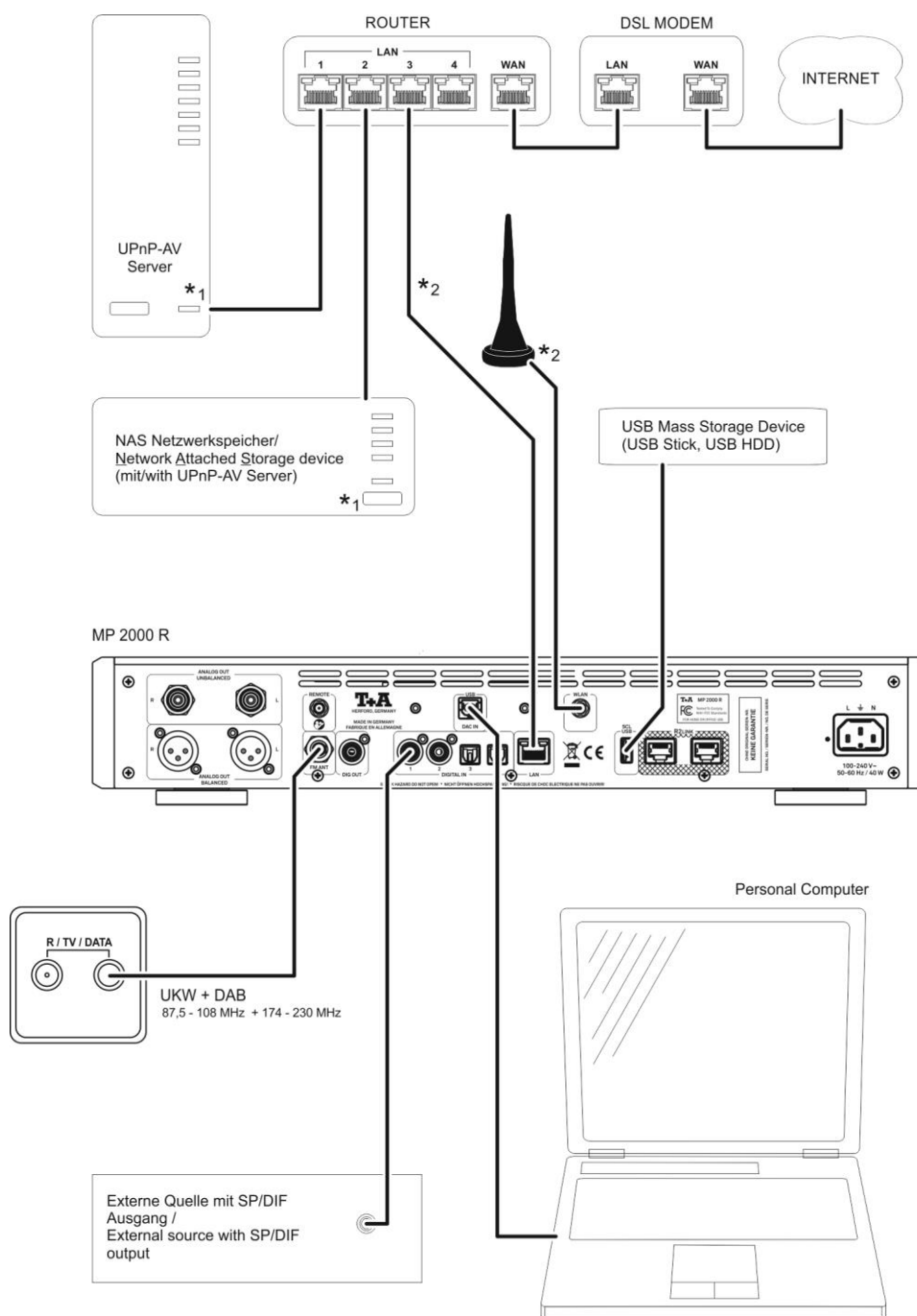
接线示意图
