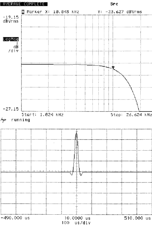
贝塞尔插值器的频率响应和瞬态特性
