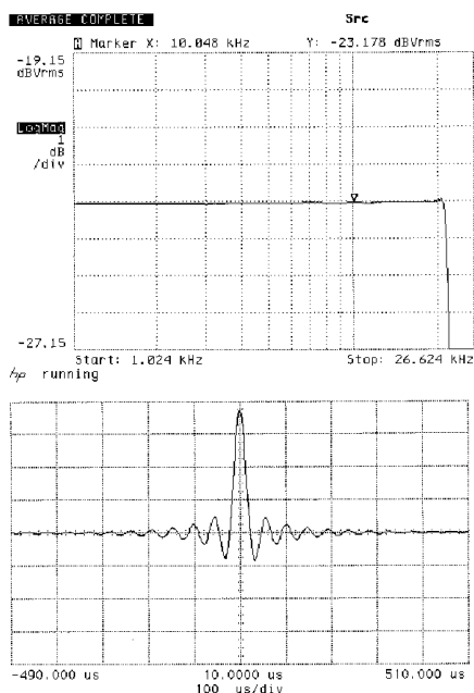
长程（有限脉冲响应）滤波器的频率响应和瞬态特性
