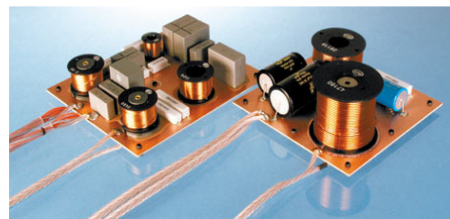
Die aufwändige FSR-Frequenzweiche der TAL X1.1
