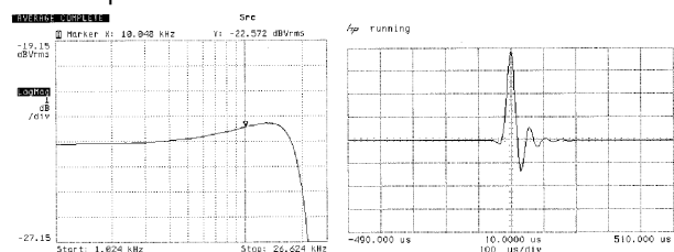
Frequenzgang und Einschwingverhalten des Bezier-Interpolators plus IIR-Filter
