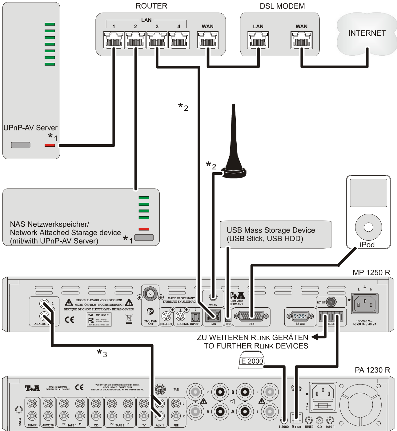
Anschluss-Schema / Wiring diagram: MP 1250 R in einer T+A Systemanlage mit R LINK Steuerung
